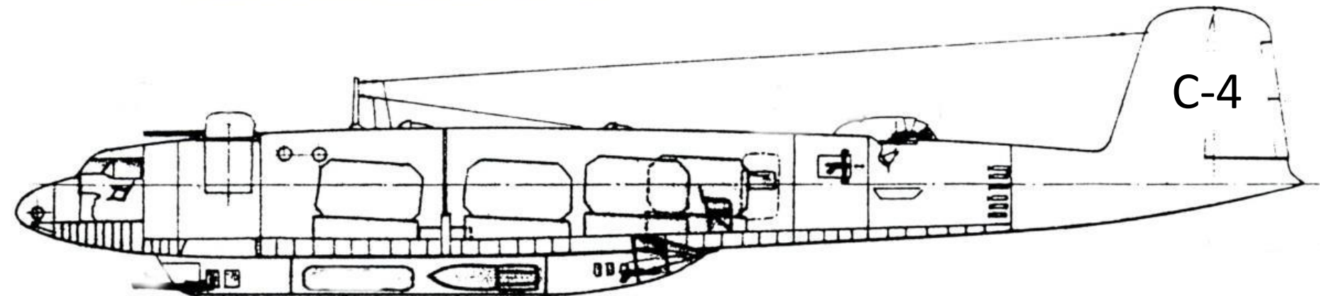
Fw 200 Rumpf: C-1, C-3 und C-4 Vergleich
